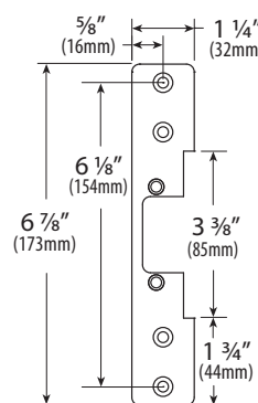
ESP3B - HOLLOW METAL DOOR
