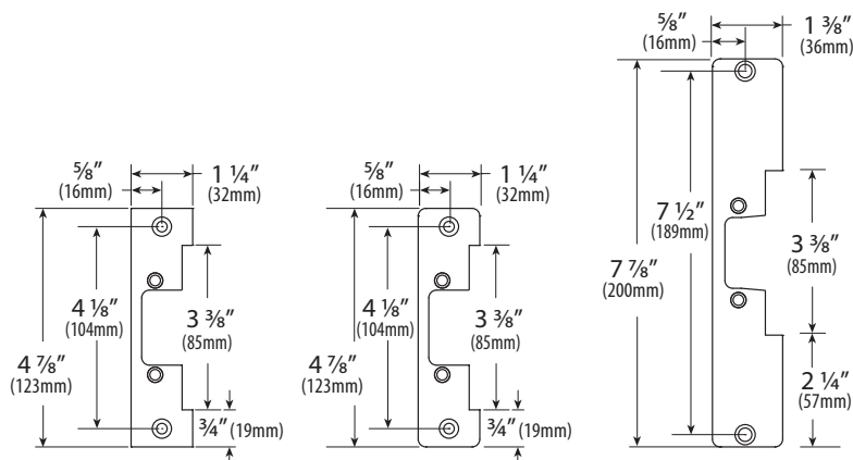
ESP1B - ANSI SQUARE
