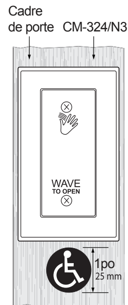
Schéma 4 Positionnement de l'autocollant handicapé
